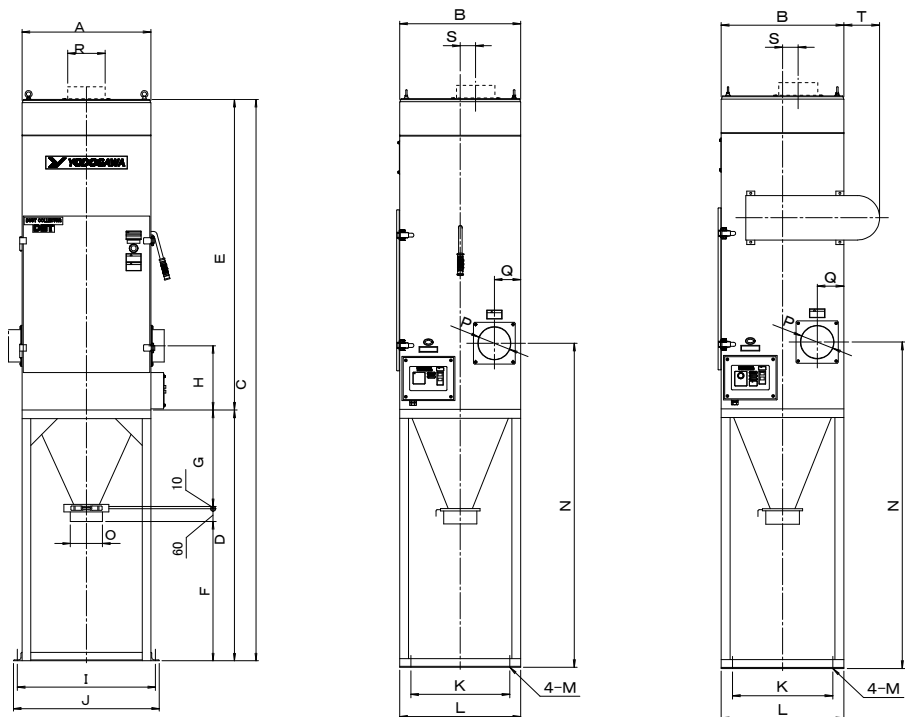
電動シェイキング装置
