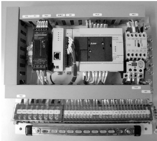
制御盤
