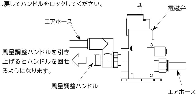
エアホース
