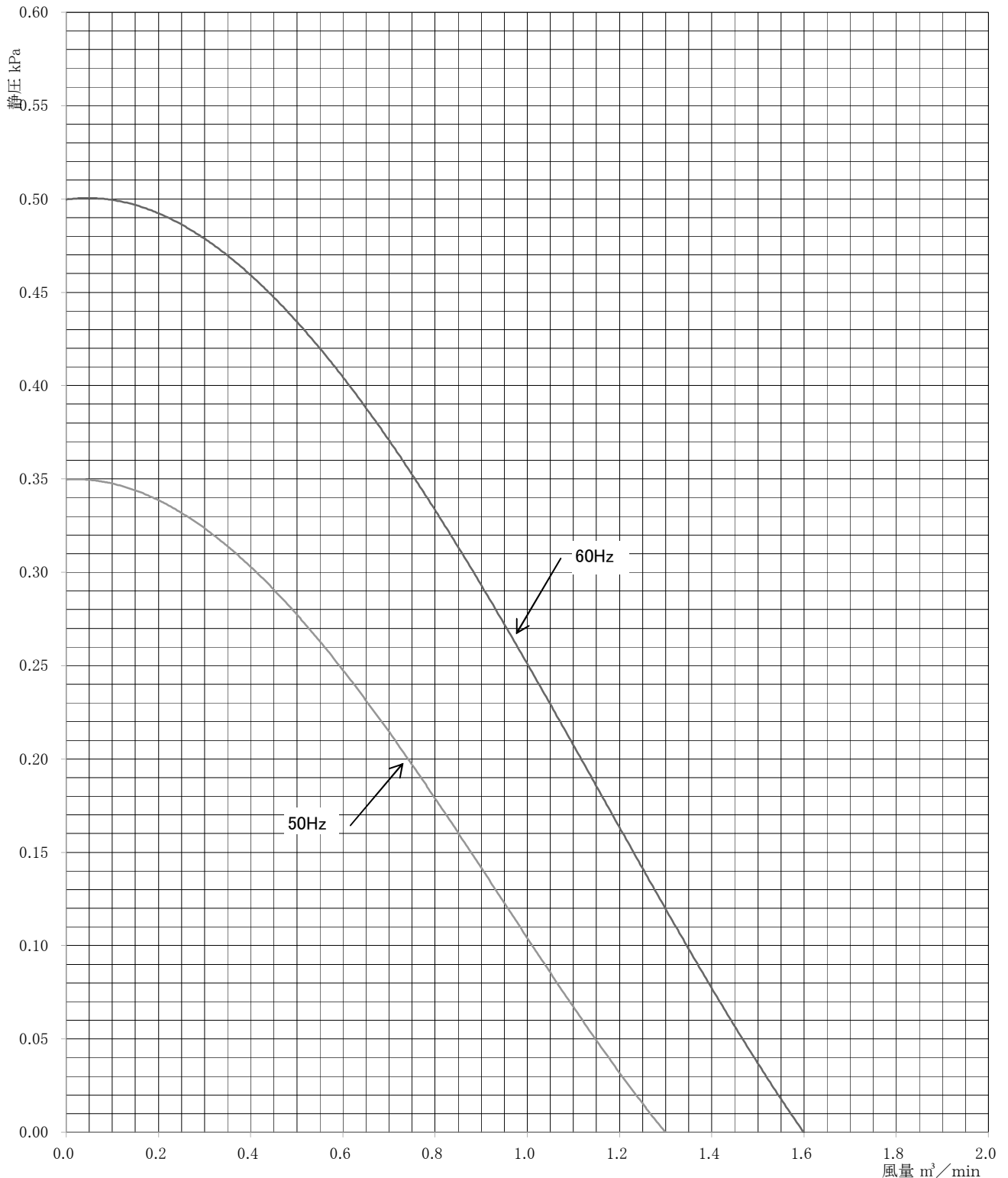
性 能 曲 線
