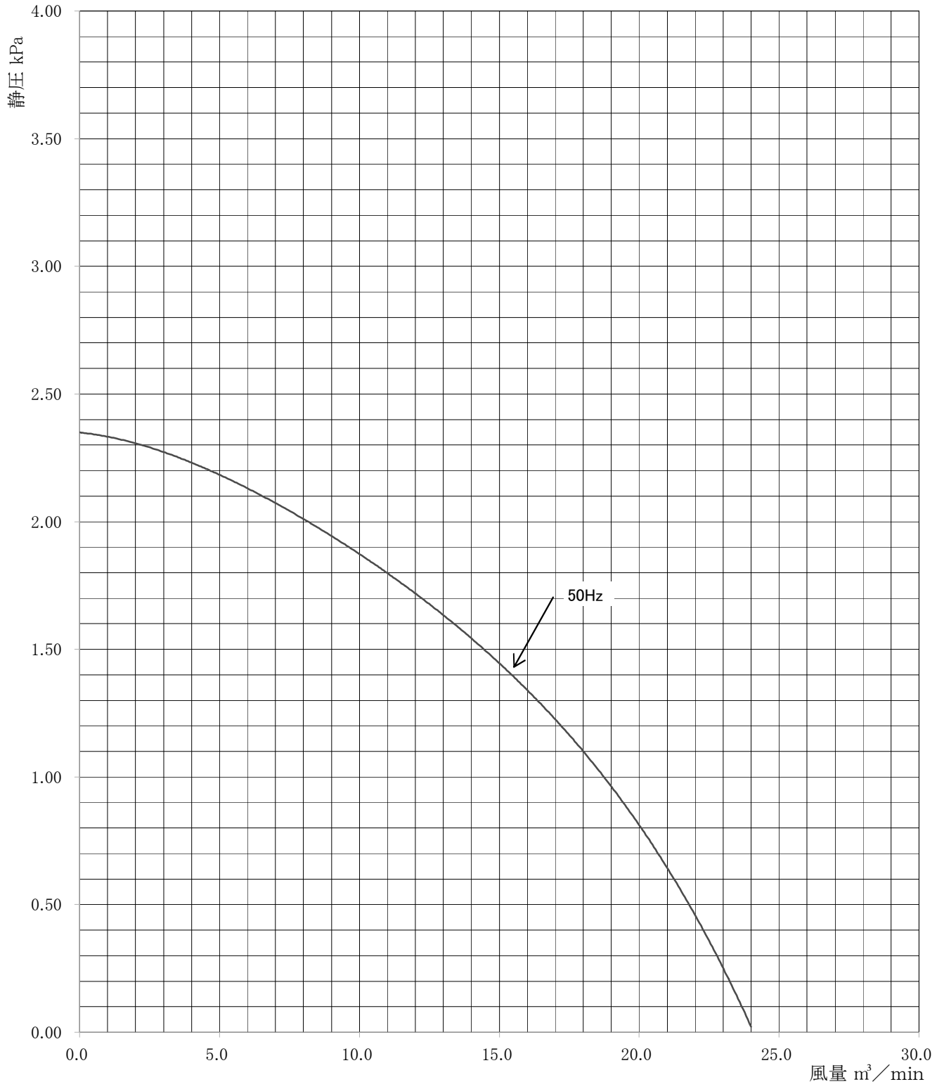
性 能 曲 線
