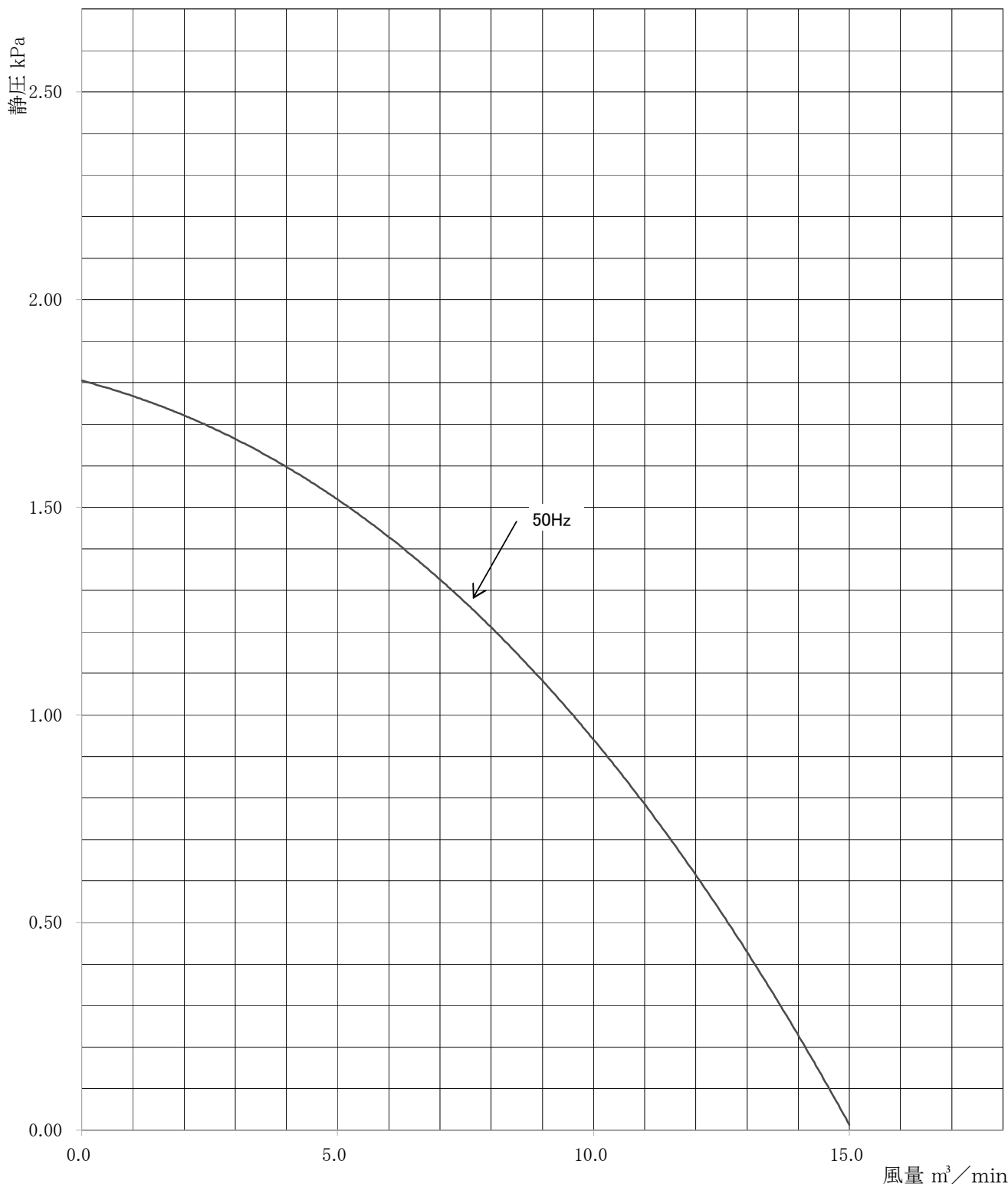
性 能 曲 線
