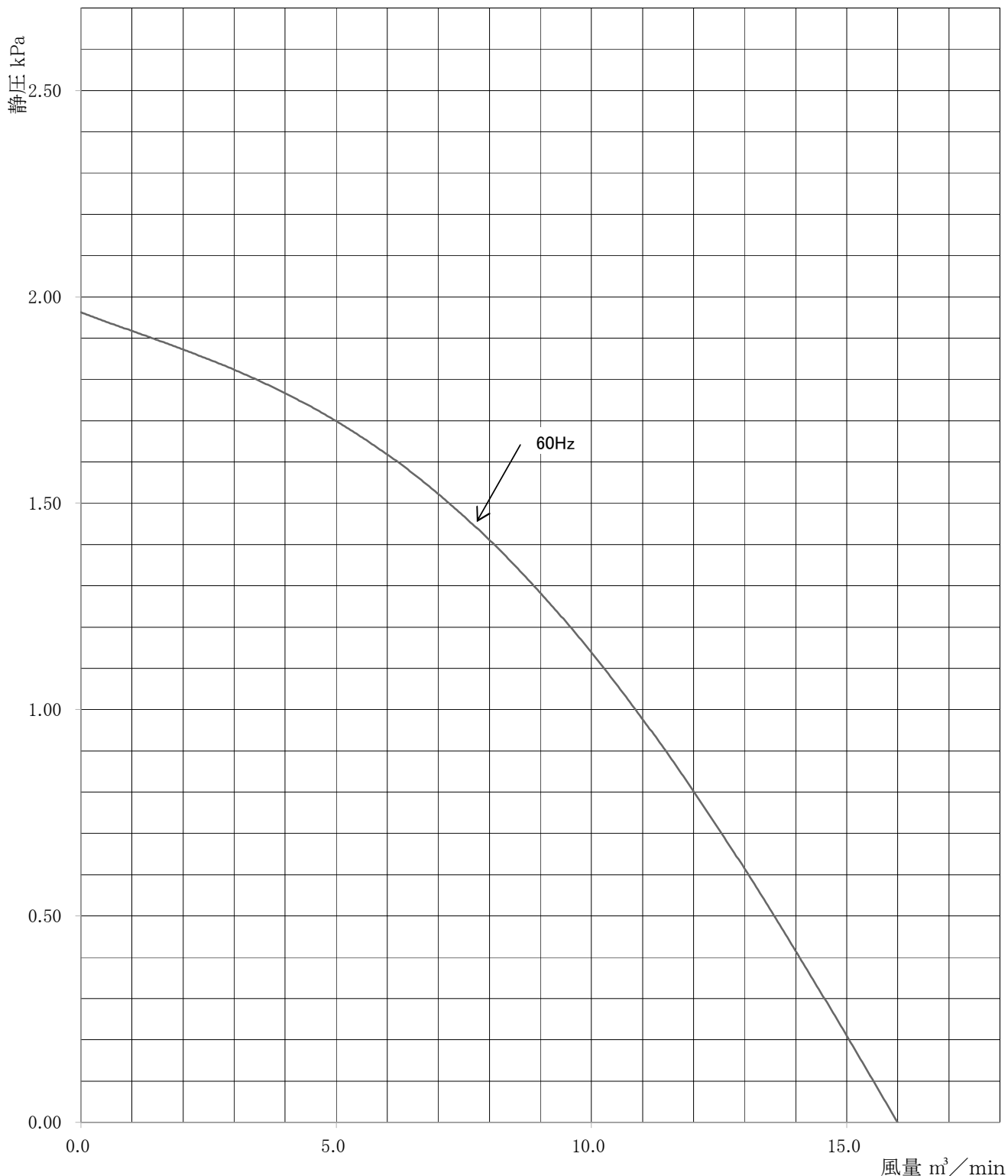
性 能 曲 線
