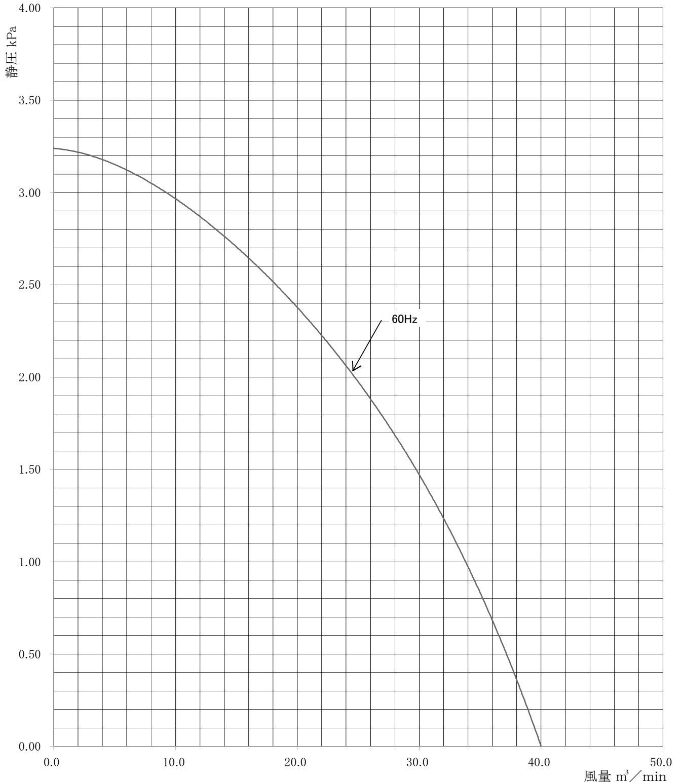
性 能 曲 線
