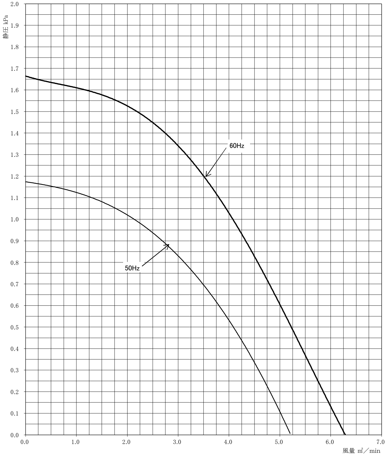
性 能 曲 線
