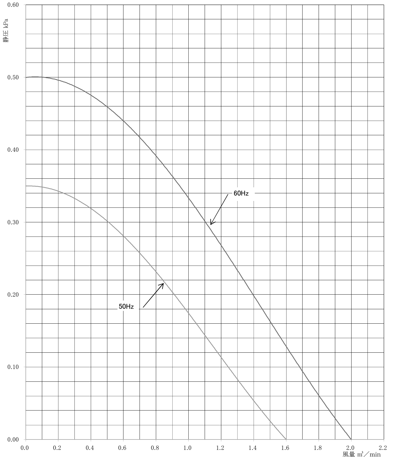
性 能 曲 線
