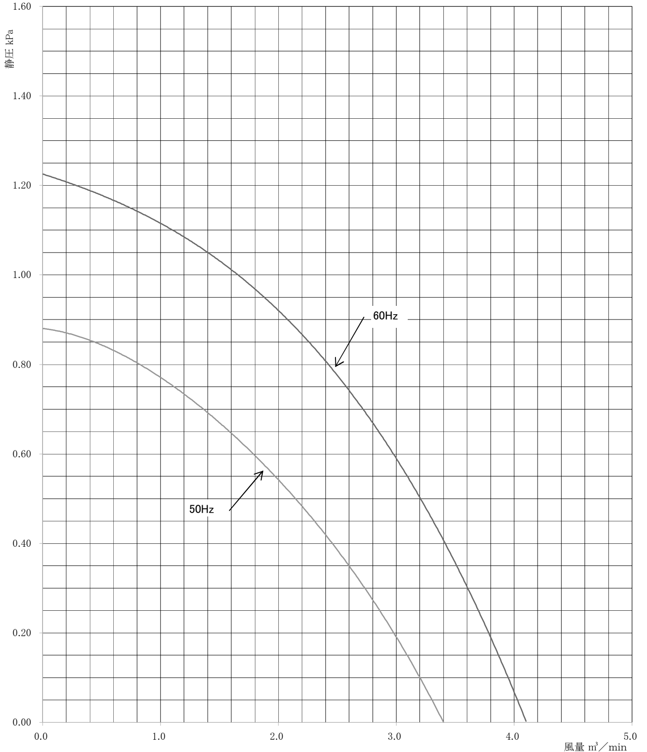
性 能 曲 線
