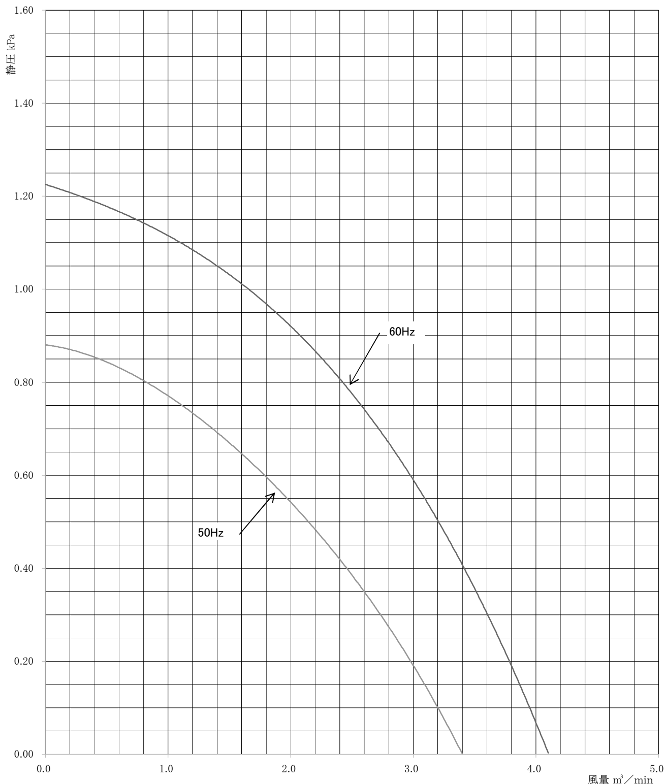
性 能 曲 線
