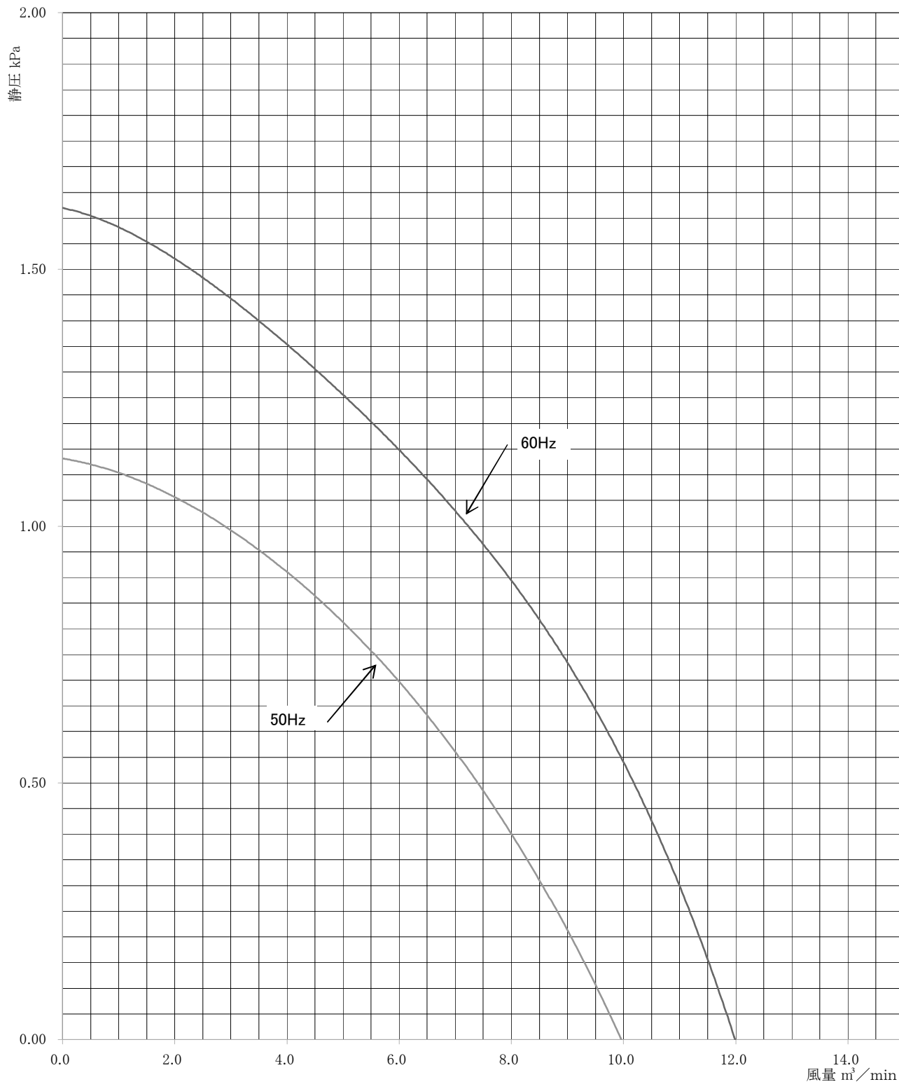
性 能 曲 線
