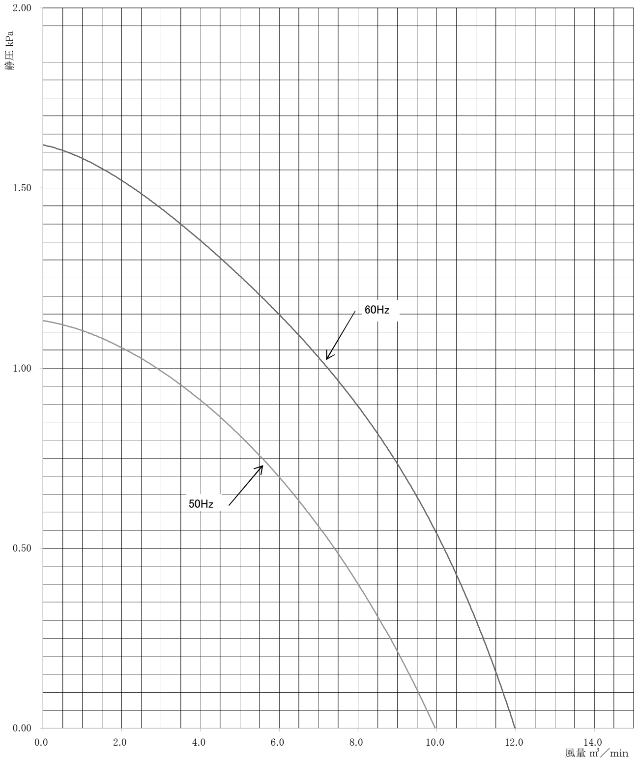
性 能 曲 線
