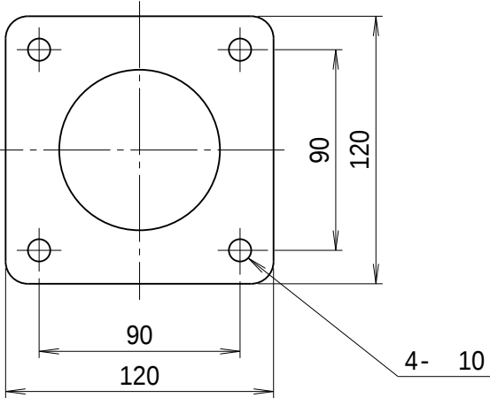
吐出し口取付寸法
