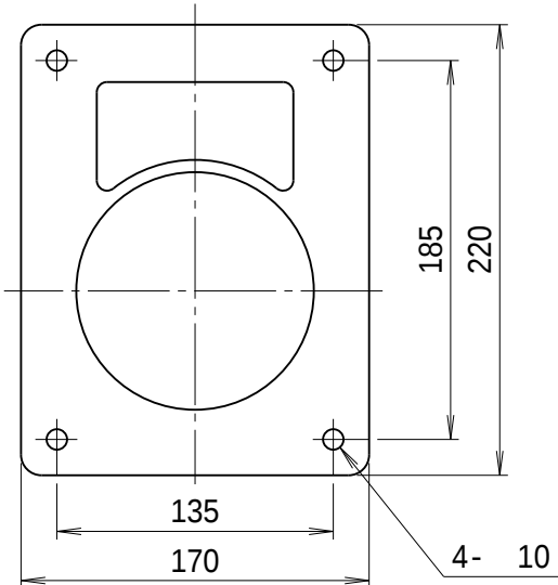
吐出し口取付寸法(1/4)
