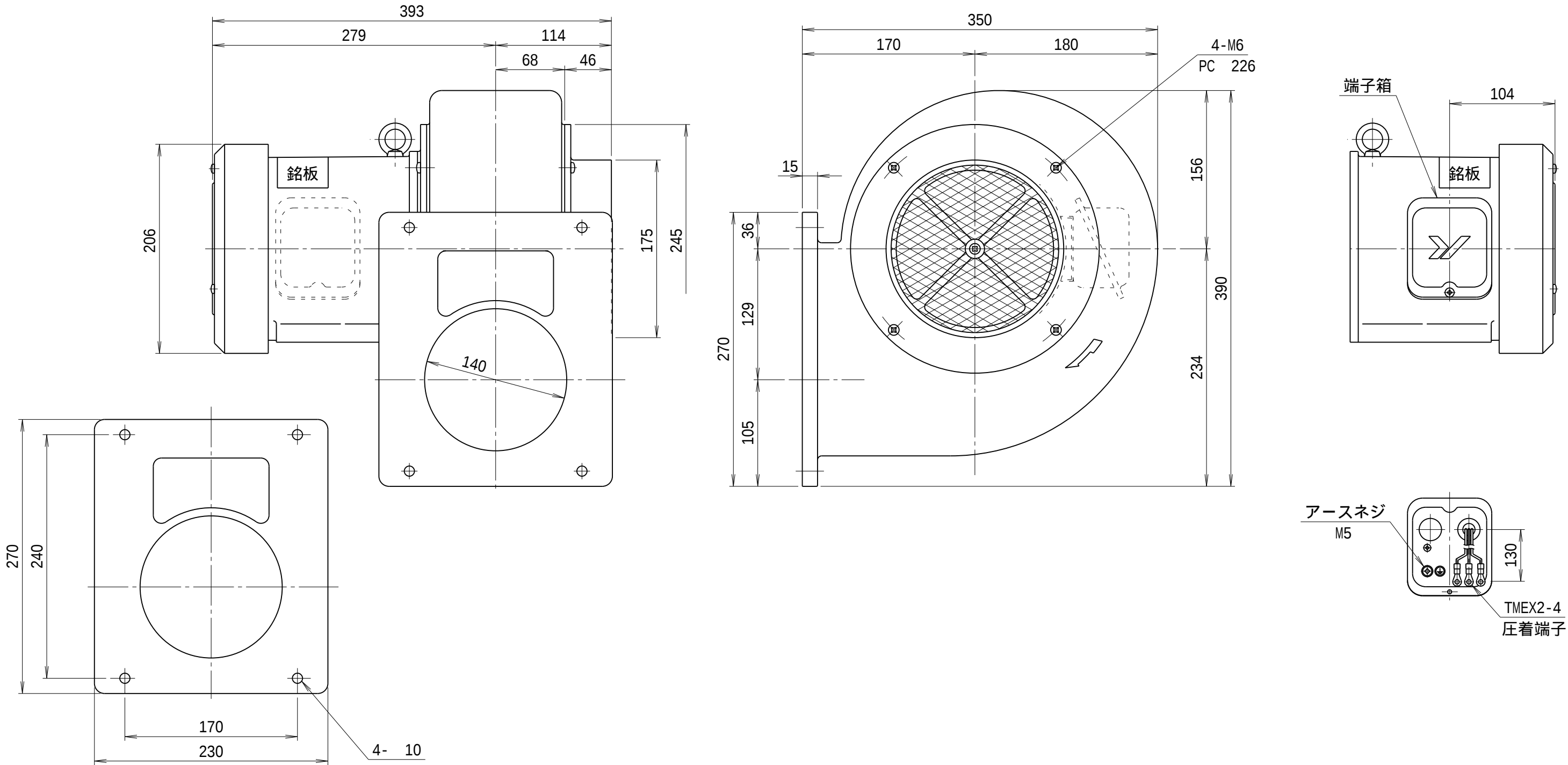
吐出し口取付寸法
