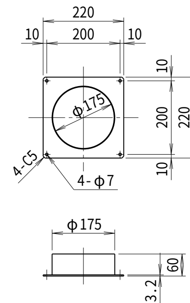
吸込口金詳細図
