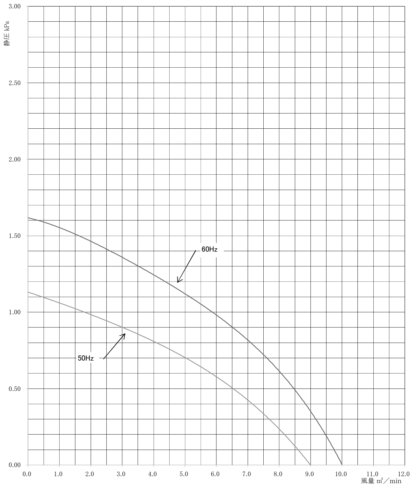
性 能 曲 線
