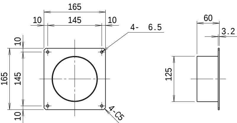
吸込口詳細図(1/6)
