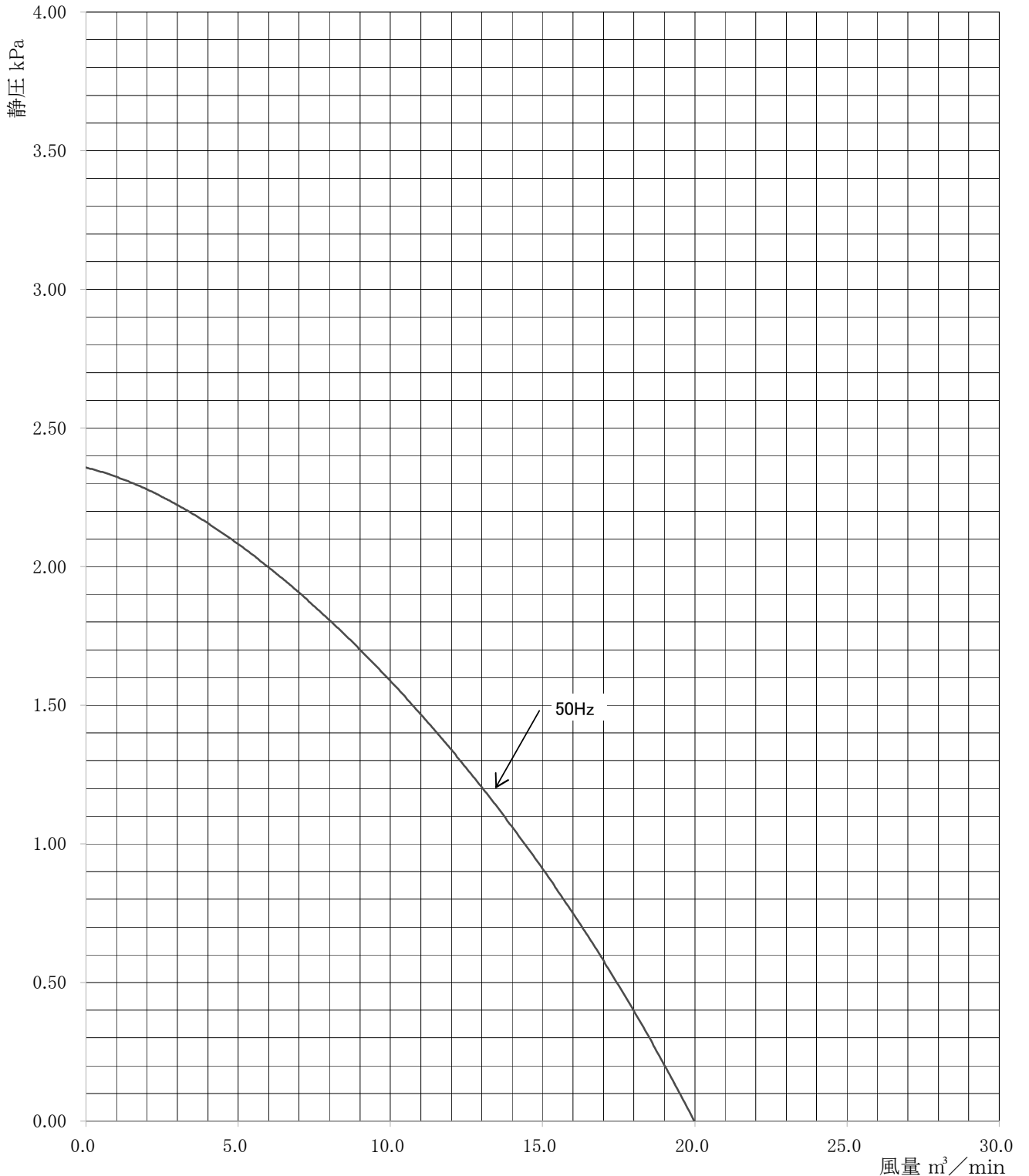
性 能 曲 線
