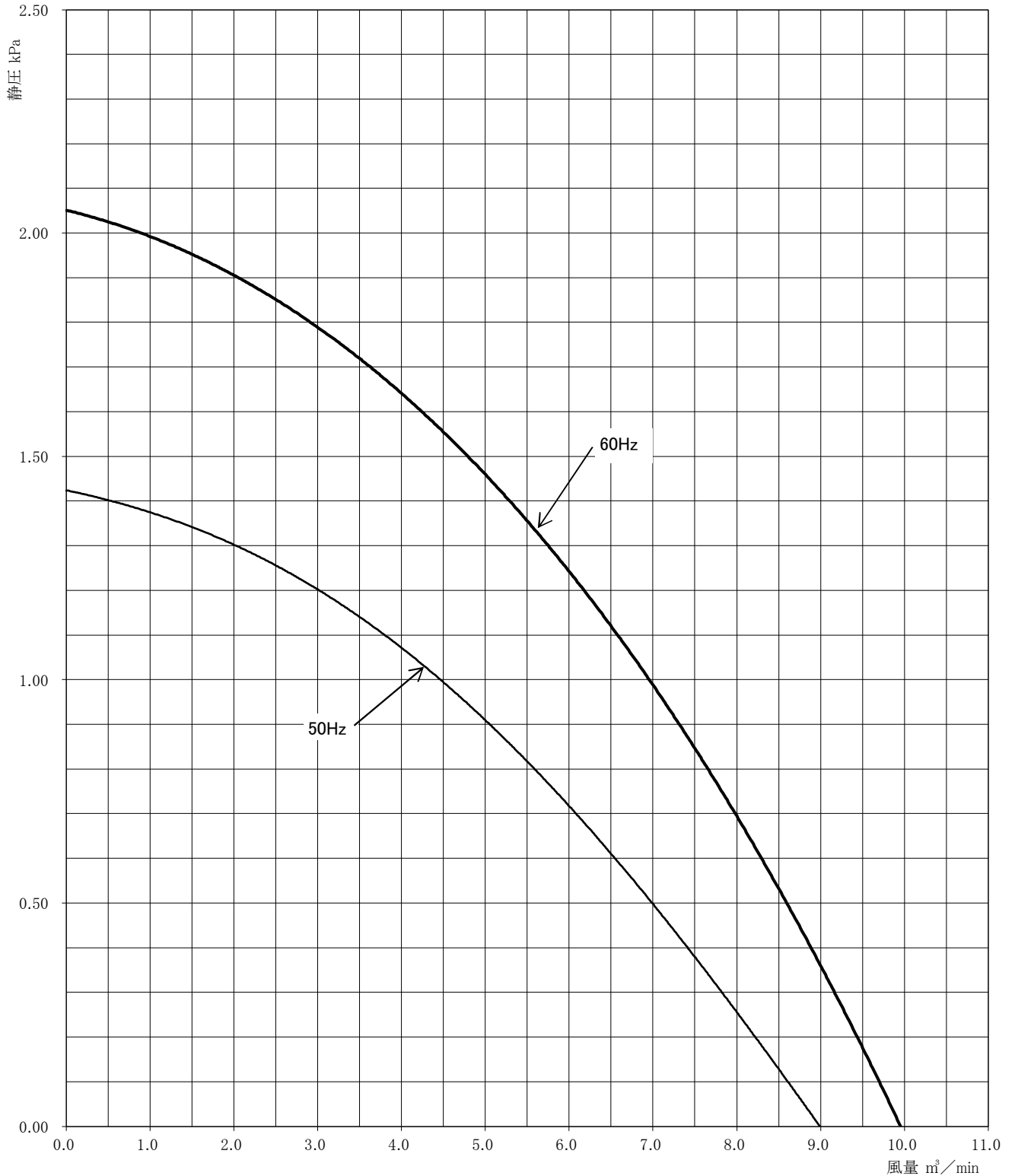
性 能 曲 線
