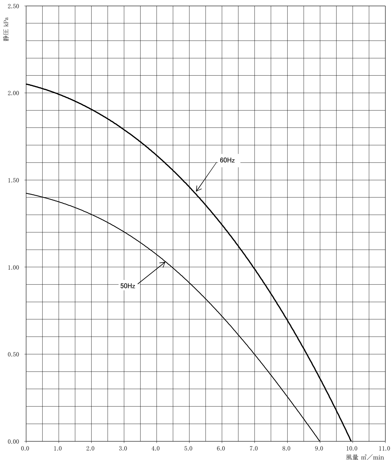
性 能 曲 線
