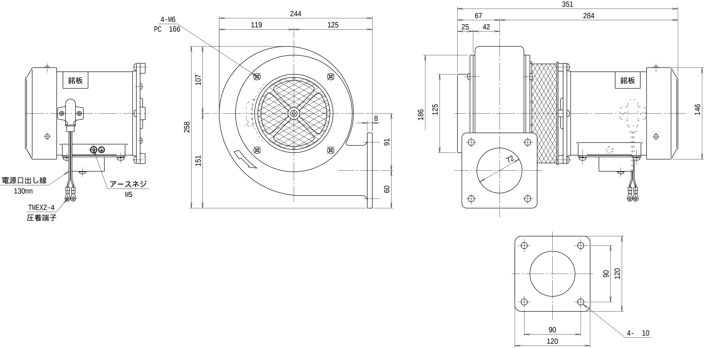
吐出し口取付寸法
