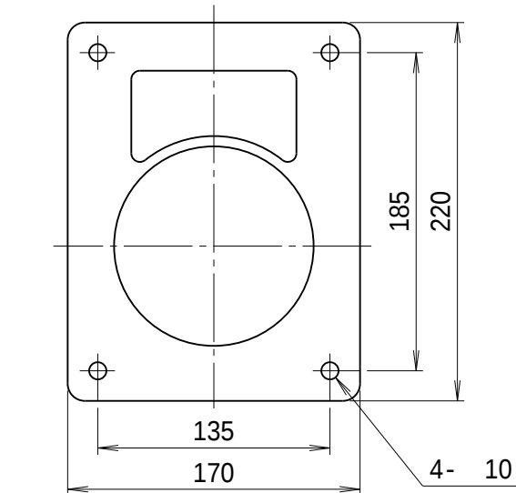
吐出し口取付寸法 (1/4)
