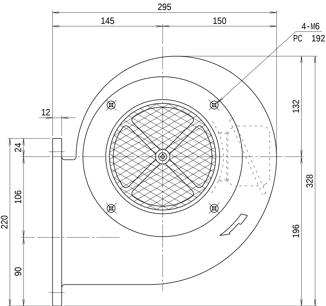
吐出し口取付寸法 (1/4)
