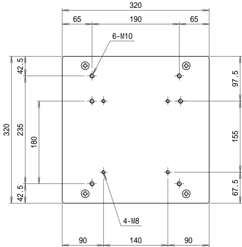
取付ピッチ詳細図(1/5)
